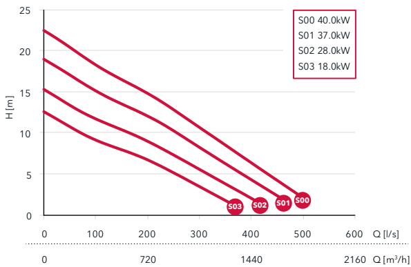
DN300
