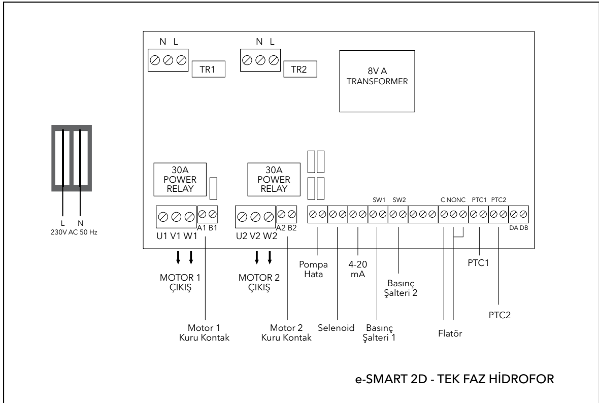
Şekil 7. e-SMART Devre Şeması - Tek Faz Hidrofor
