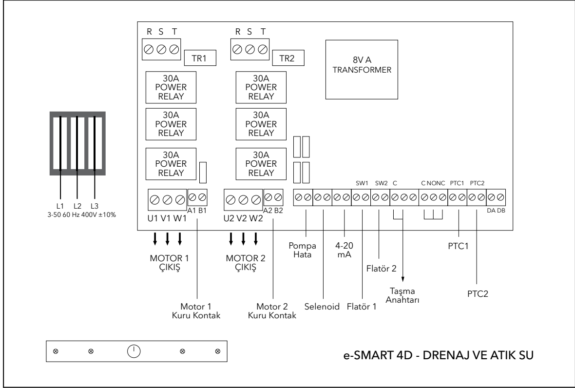
Şekil 6. e-SMART Devre Şeması - Drenaj ve Atık Su
