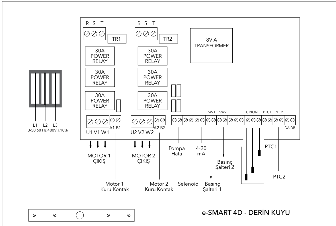
Şekil 5. e-SMART Devre Şeması - Derin Kuyu
