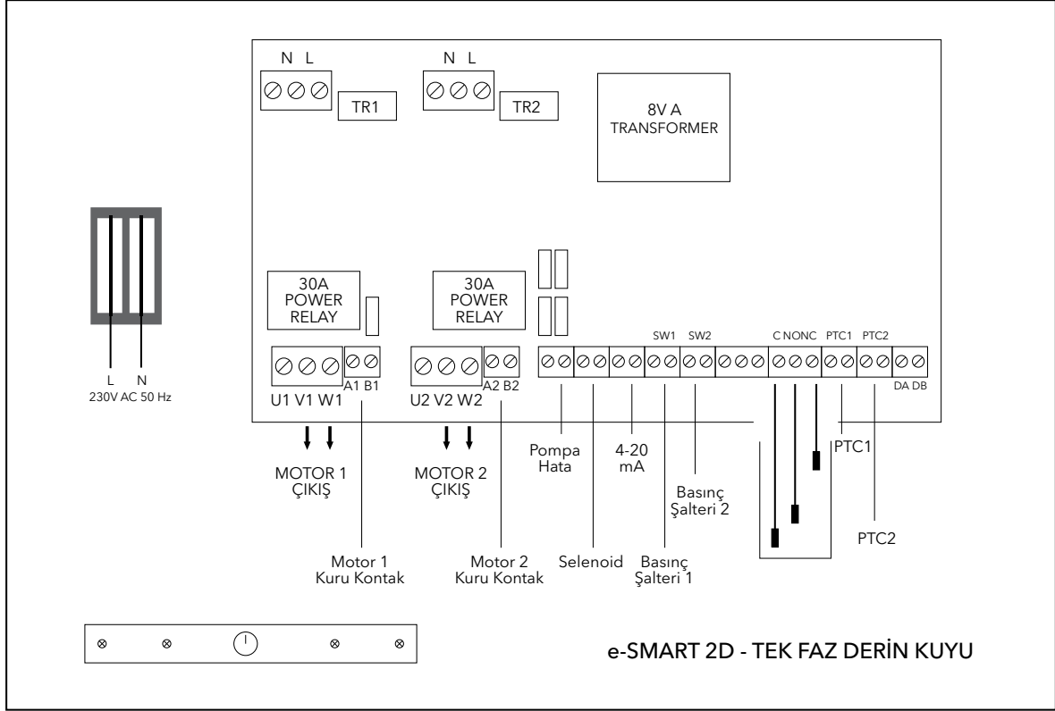
Şekil 8. e-SMART Devre Şeması - Tek Faz Derin Kuyu
