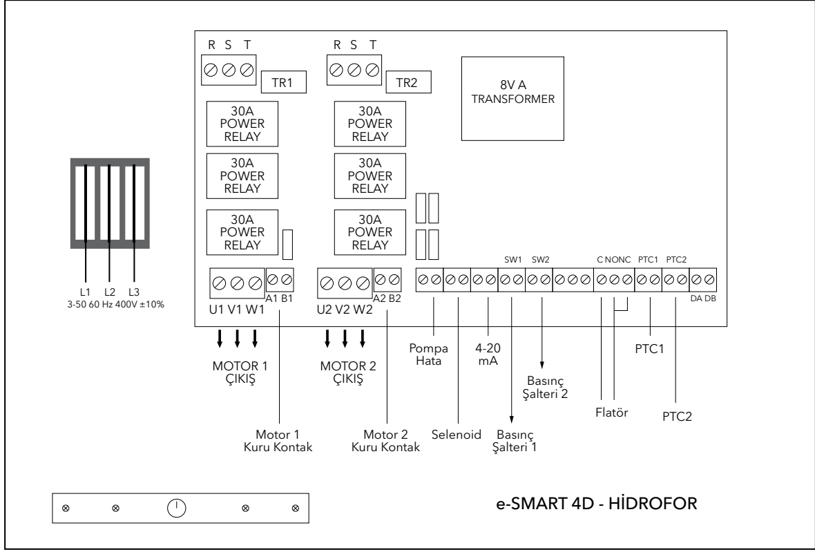
Şekil 4. e-SMART Devre Şeması - Hidrofor
