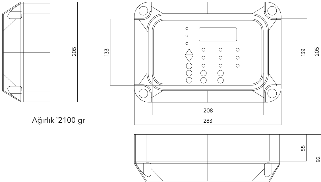
Şekil 3. Panel Boyutları
