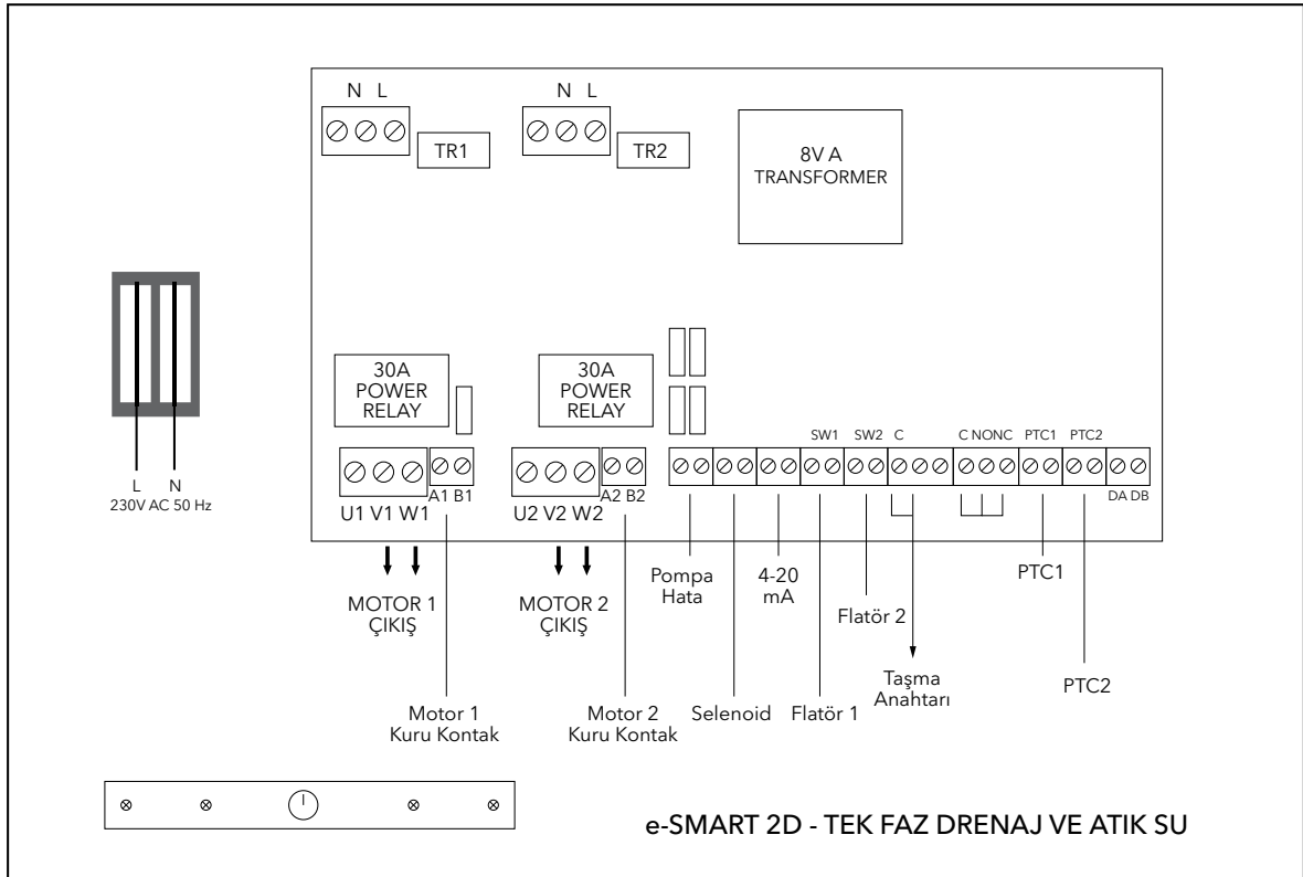
Şekil 9. e-SMART Devre Şeması - Tek Faz Drenaj ve Atık Su
